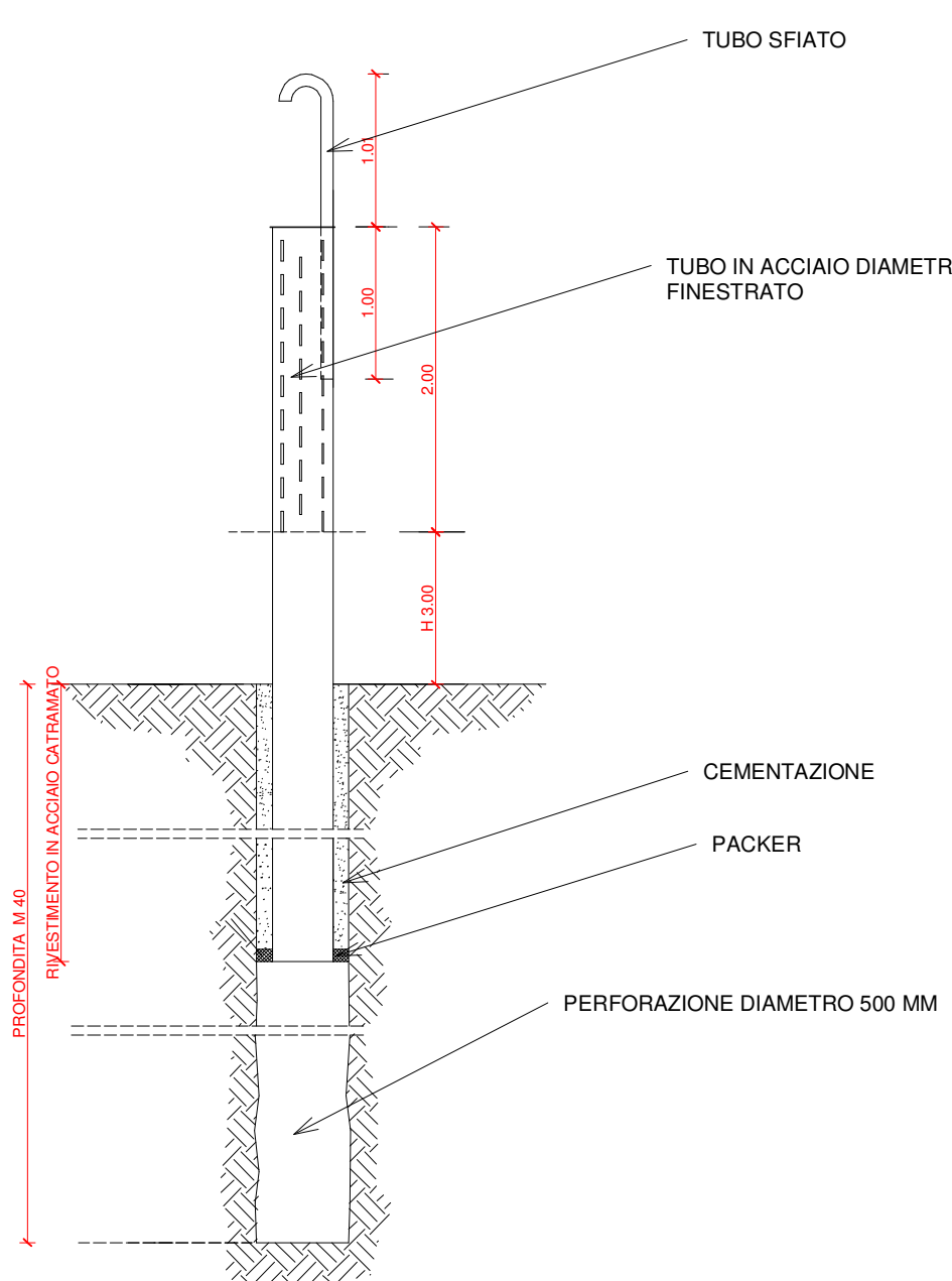
5 PARTICOLARE POZZO ANIDRO TAV.5 1 : 50
