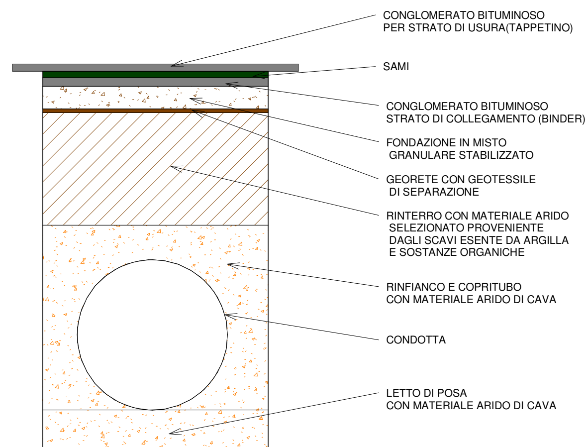
6 PARTICOLARE SCAVO TAV.5 1 : 20
