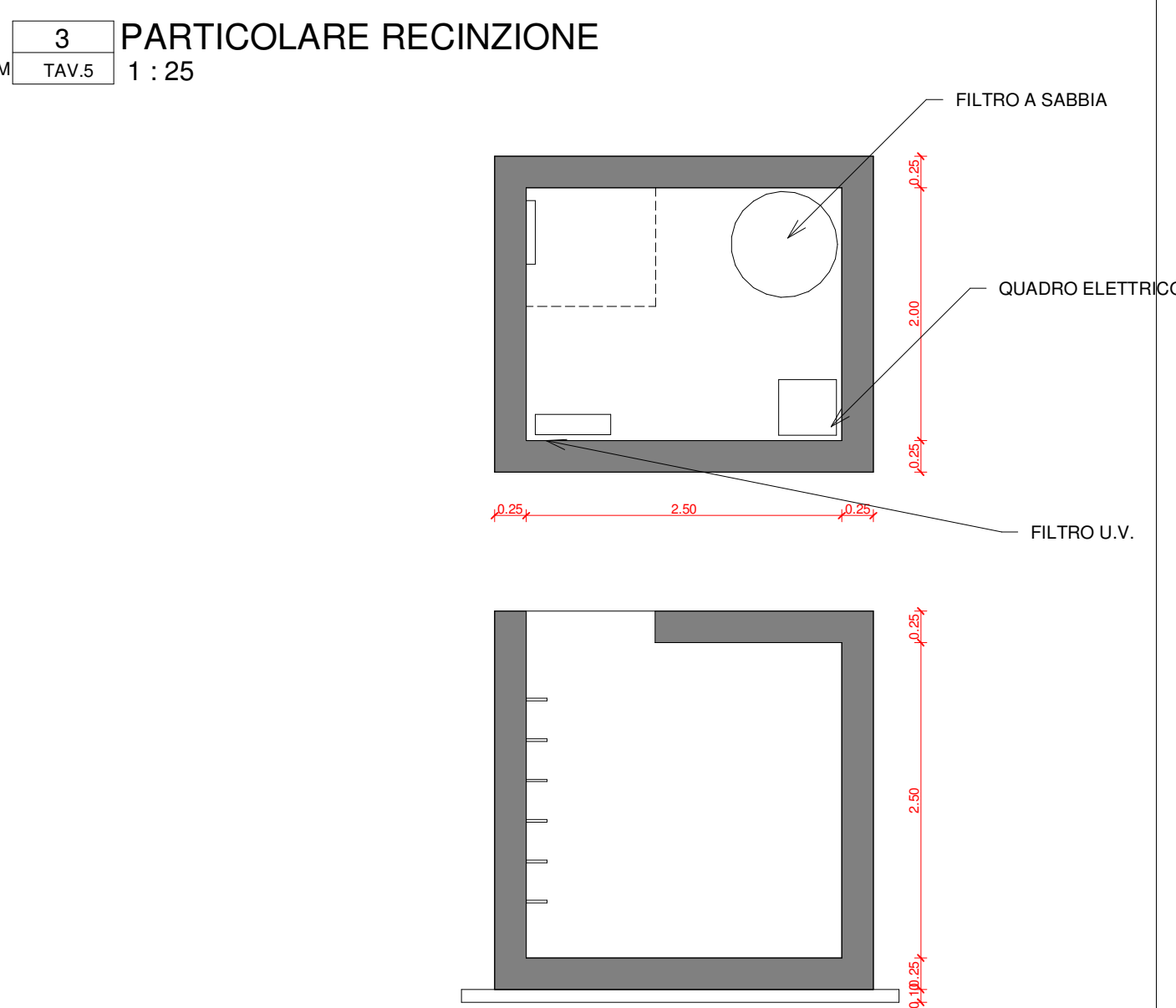
4 VANO TECNICO AFFINAMENTO TAV.5 1 : 50
