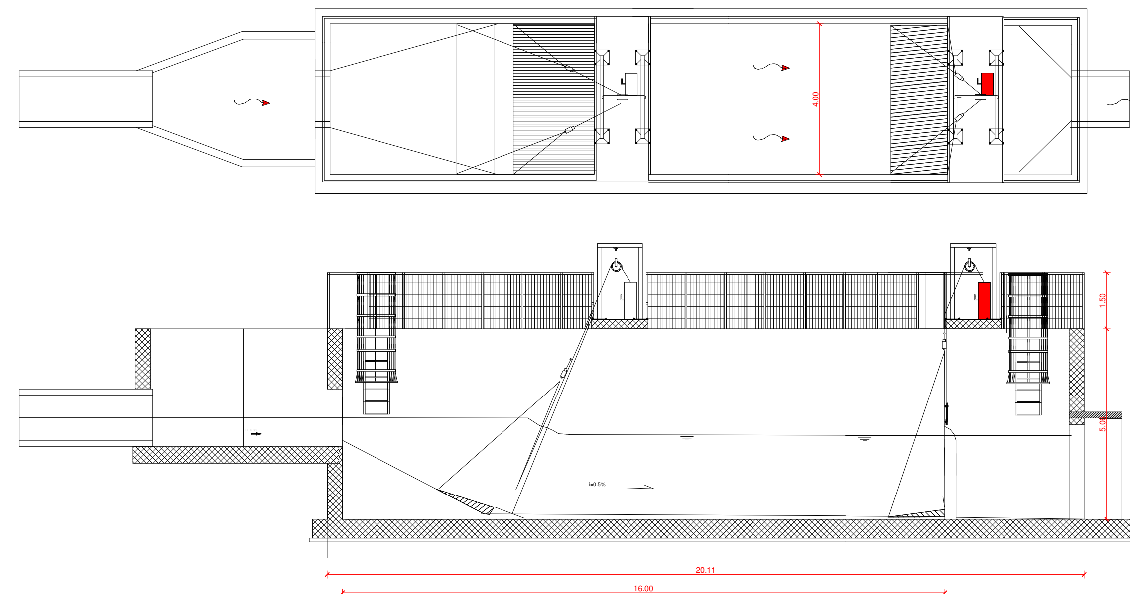
2 VASCA TRATTAMENTO ACQUE TAV.5 1 : 100
